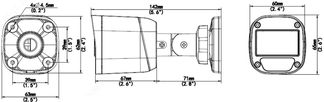
UAC-B115-F28/F40-W
